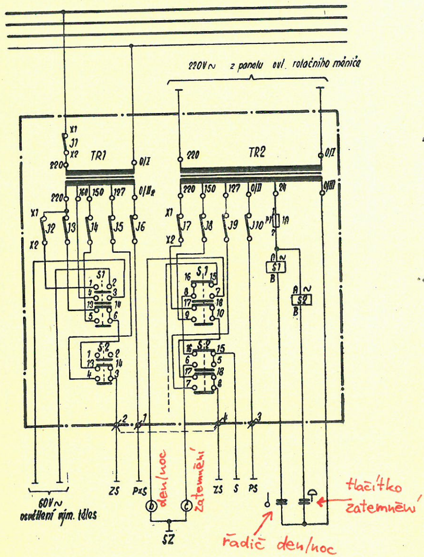
Obr. 269. Schéma zapojení panelu pro napájení návštěvidel
