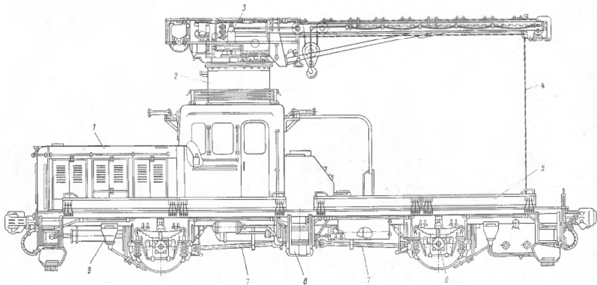
Рис. 10.14. Грузовая авторезина ДГК-5
